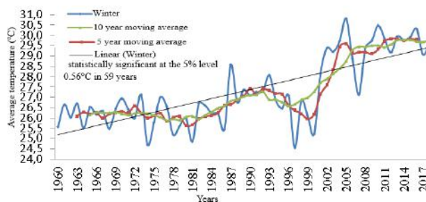
Figura 5. Tendência linear da temperatura média anual e estacional, seguidamente das médias móveis de 5 e 10 anos da estação inverno no município de Bom Jesus do Piauí no período 1960-2018.
