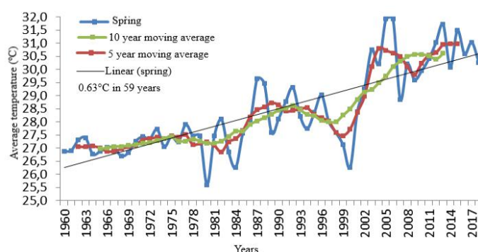
Figura 7. Tendência linear da temperatura média anual e estacional, seguidamente das médias móveis de 5 e 10 anos na estação primavera no município de Bom Jesus do Piauí no período 1960-2018.
