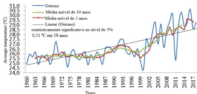
Figura 4. Tendência linear da temperatura anual e estacional, seguidamente das médias móveis de 5 e 10 anos da estação outono no município de Bom Jesus do Piauí no período 1960-2018.
