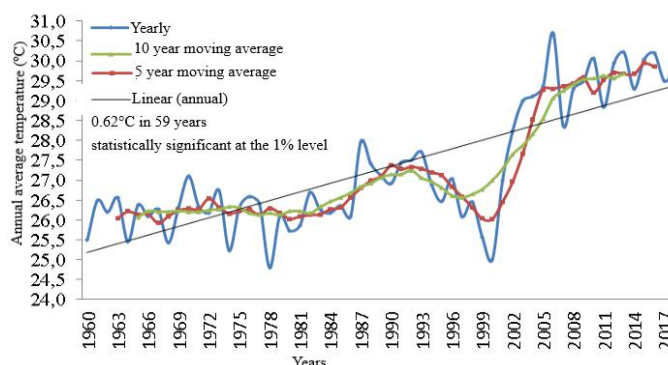
Figura 2. Representação da temperatura anual e estacional, seguidamente das médias móveis de 5 e 10 anos no município de Bom Jesus do Piauí no período 1960-2018.
