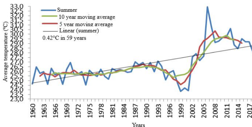
Figura 6. Tendência linear da temperatura média do ar anual e estacional, seguidamente das médias móveis de 5 e 10 anos da estação verão no município de Bom Jesus do Piauí no período 1960-2018.
