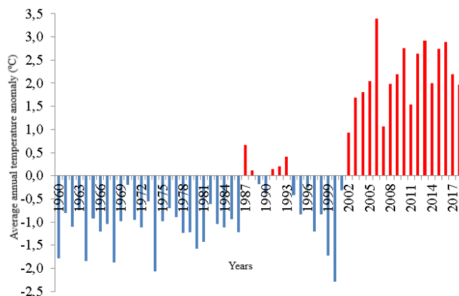
Figura 3. Variabilidade da anomalia da temperatura anual e estacional, no município de Bom Jesus do Piauí no período 1960-2018.
